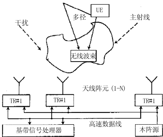
图1 CDMA 基地站的示意图
