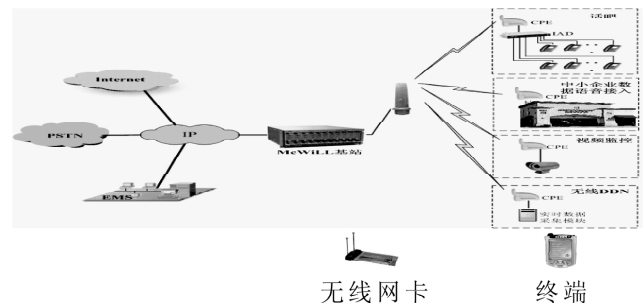
图2 McWiLL 宽带无线接入系统示意图
