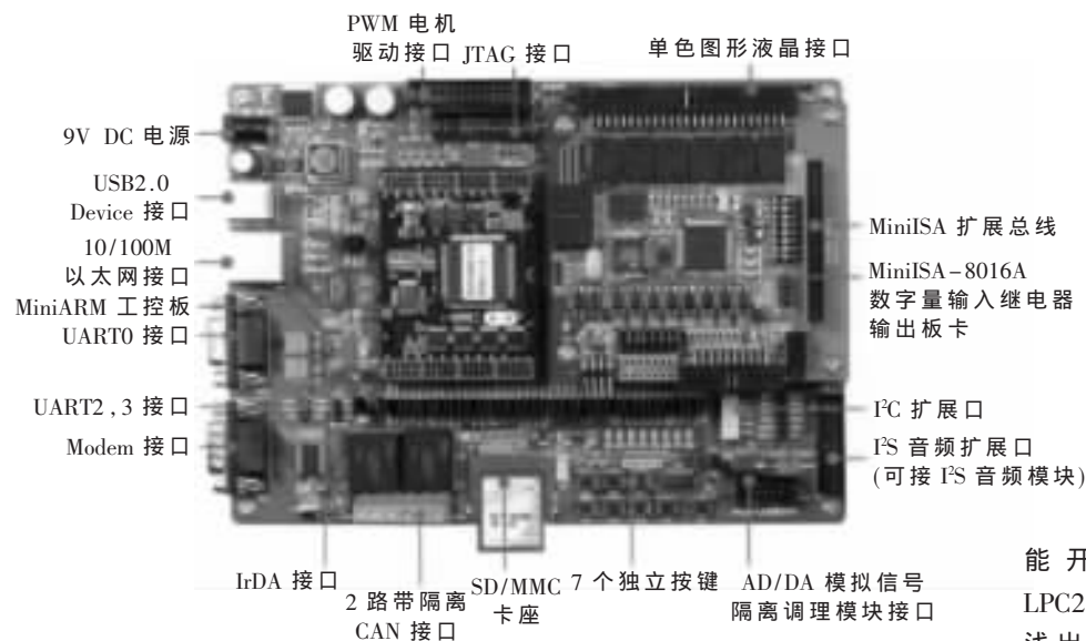
图 1 SmartARM2300 通用教学/竞赛/工控开发平台
