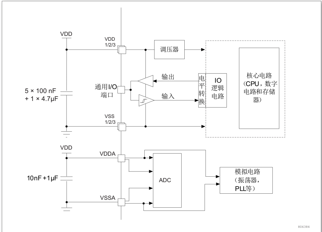
图 9. 供电方案
