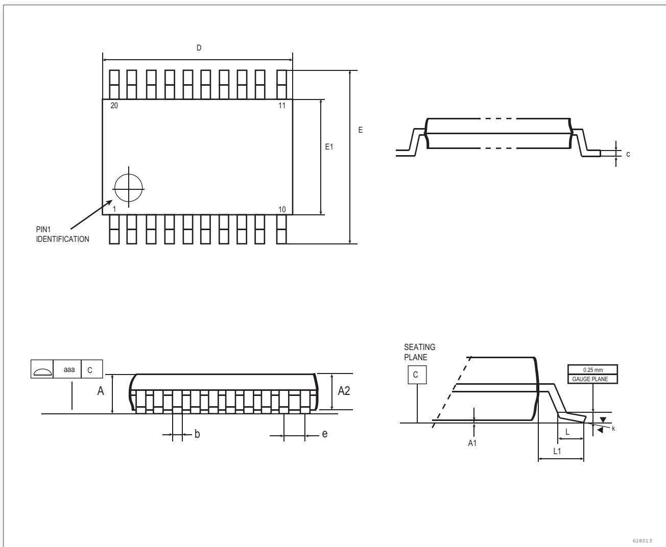
图 24. TSSOP20, 20 脚低剖面长方形扁平封装图
